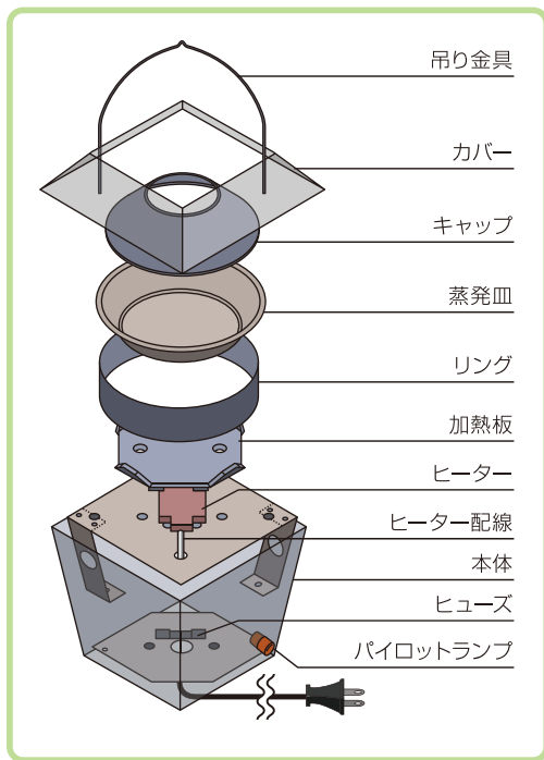
アグリ・トップ硫黄くん煙器の構造
